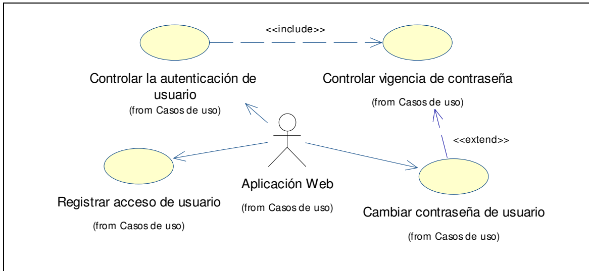
Figura 2.7 Diagrama de casos de uso del paquete Servicios.
