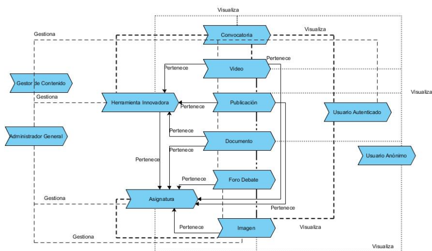
Figura 2.1. Estructura de la propuesta de solución (Elaboración propia)
