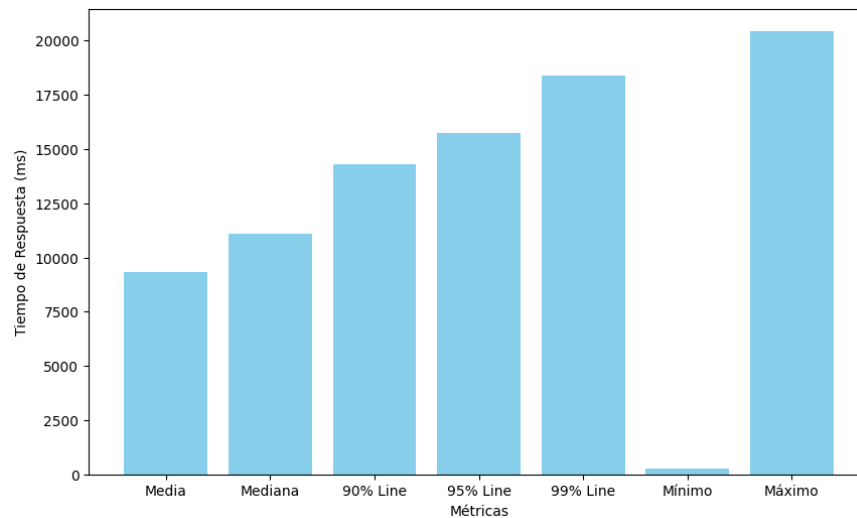
Figura 3.1. Primera Iteración de Prueba de rendimiento con la herramienta Apache Jmeter (Elaboración propia)
