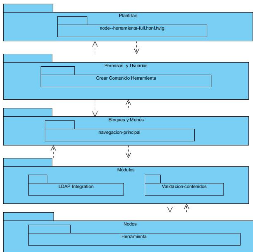
Figura 2.2. Diseño arquitectónico de la propuesta de solución (Elaboración propia)
