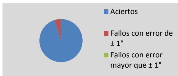
Gráfico 3.4. Total de aciertos y fallos generados por el algoritmo propuesto. De un total de 11600 imágenes, se obtuvieron 11069 aciertos (95,42%), 514 fallos en los que el error fue de \mp 1^{\circ} (4,43%), y 17 fallos en los que el error fue superior a \mp 1^{\circ} (0,15%).
