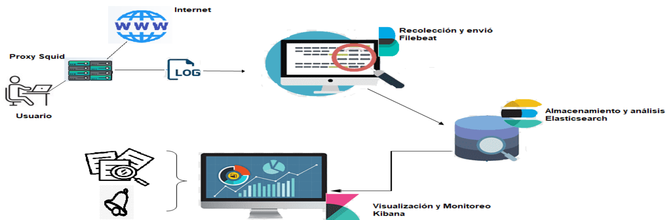
Figura 3 Arquitectura de despliegue
